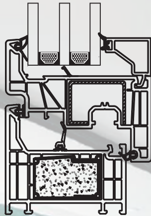
HOJA COPLANAR Uf = 0,93 W/m2K
