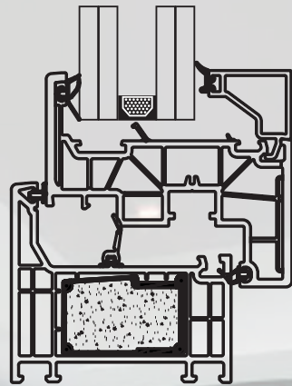
HOJA THERMOFIBRA Uf = 0,86 W/m2K
