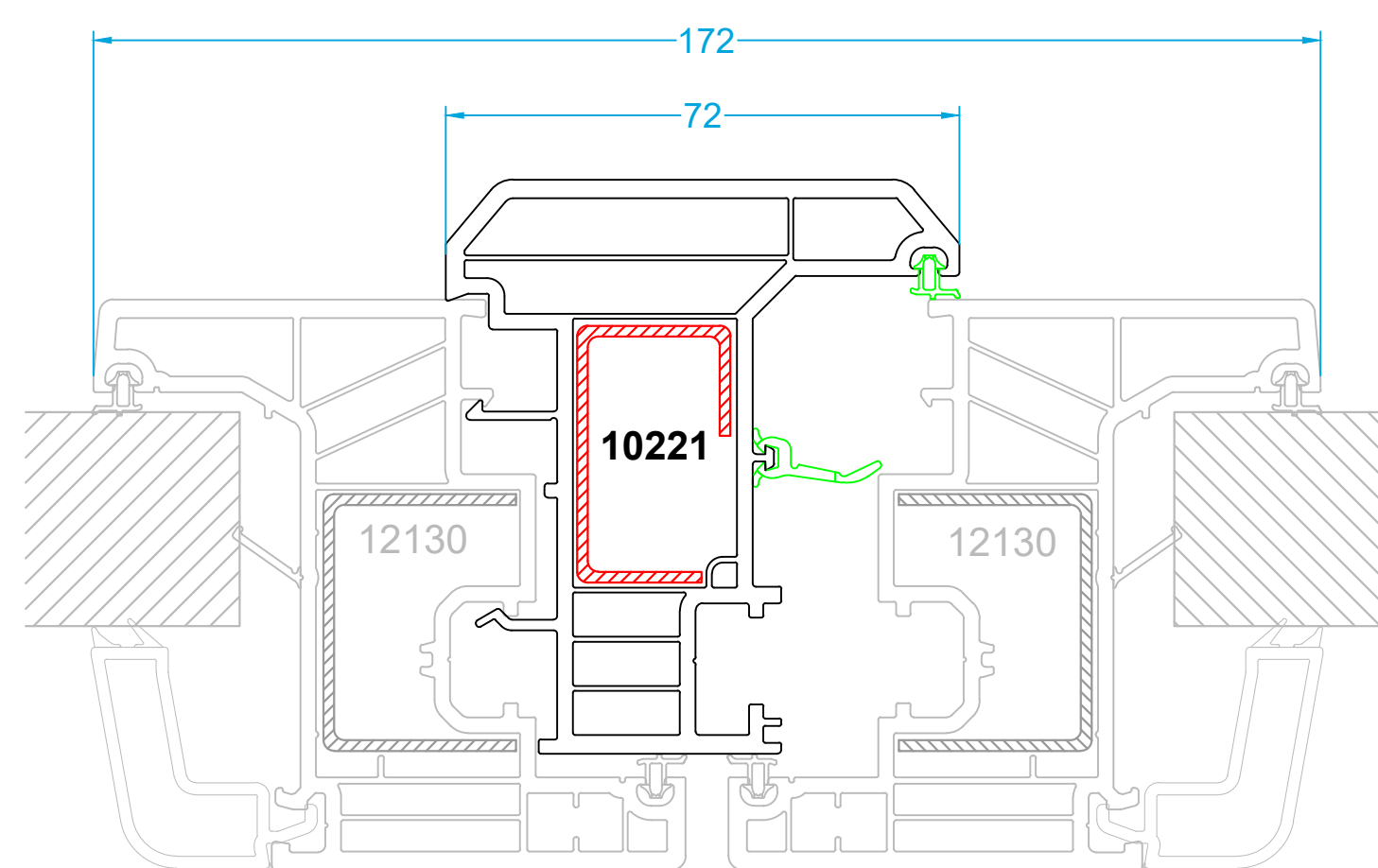
Union hojas e inversora
