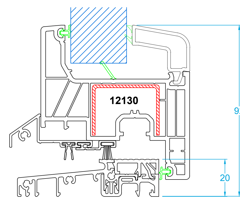
Solera de aluminio Hoja de ventana
