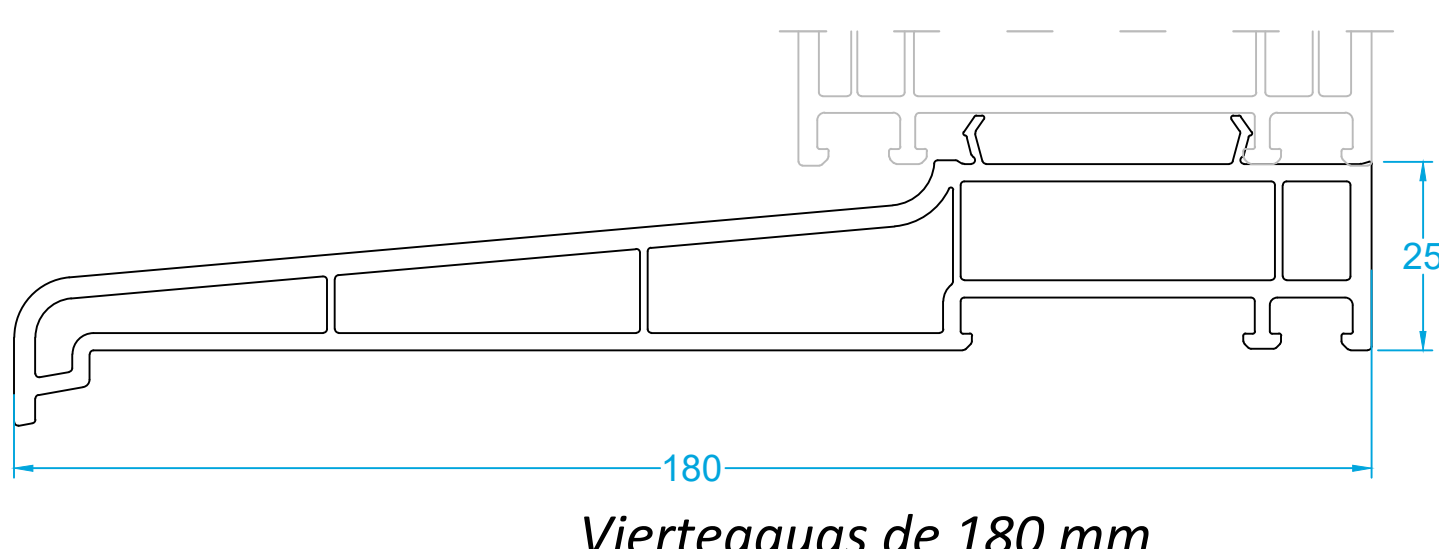
Vierteaguas de 180 mm
